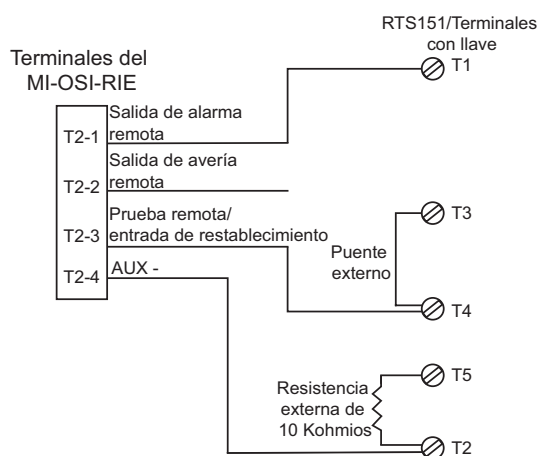
Figura 3-12: Diagrama de cableado
