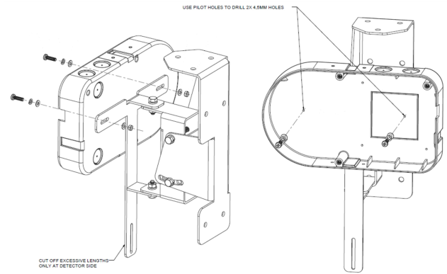
Figura 3-10: Instrucciones de montaje del detector
