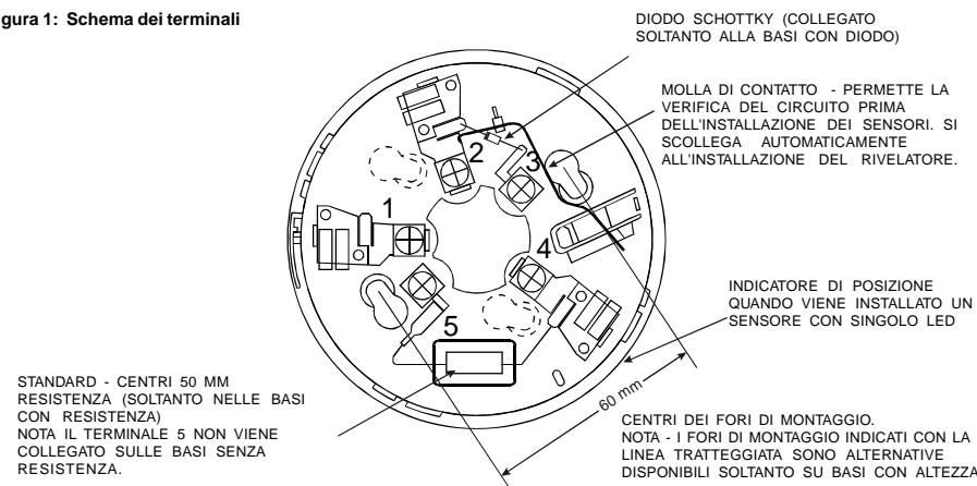
Figura 1: Schema dei terminali
