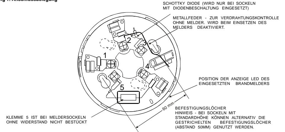
Abbildung 1: Anschlussbelegung
